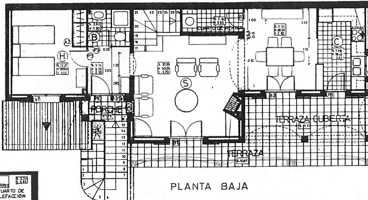
PLANTA PISO
